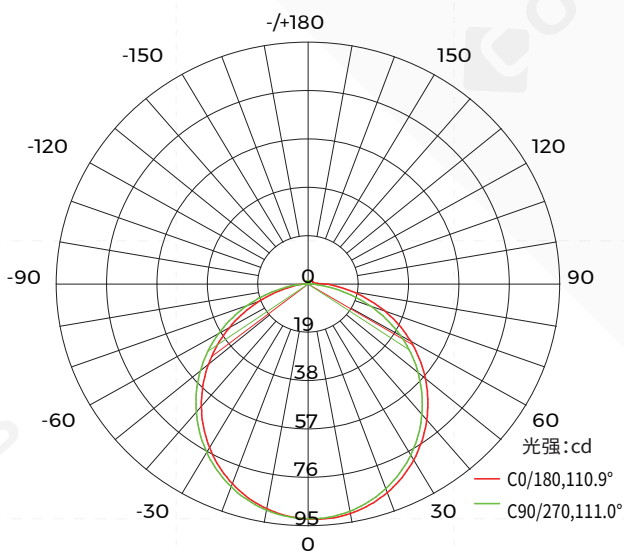
配光曲线
